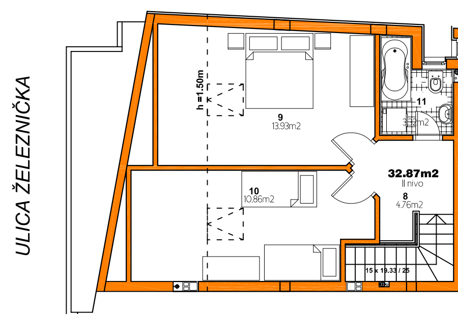
OSNOVA POTKROVLJA II NIVO, STAN BR.33
